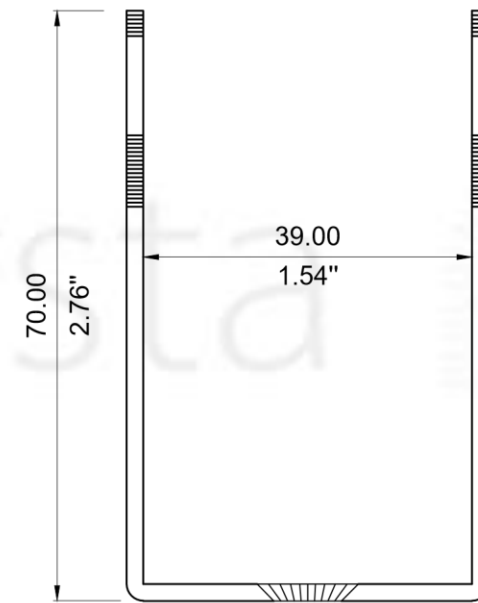
3 FRONT ELEVATION U-3 N.T.S
